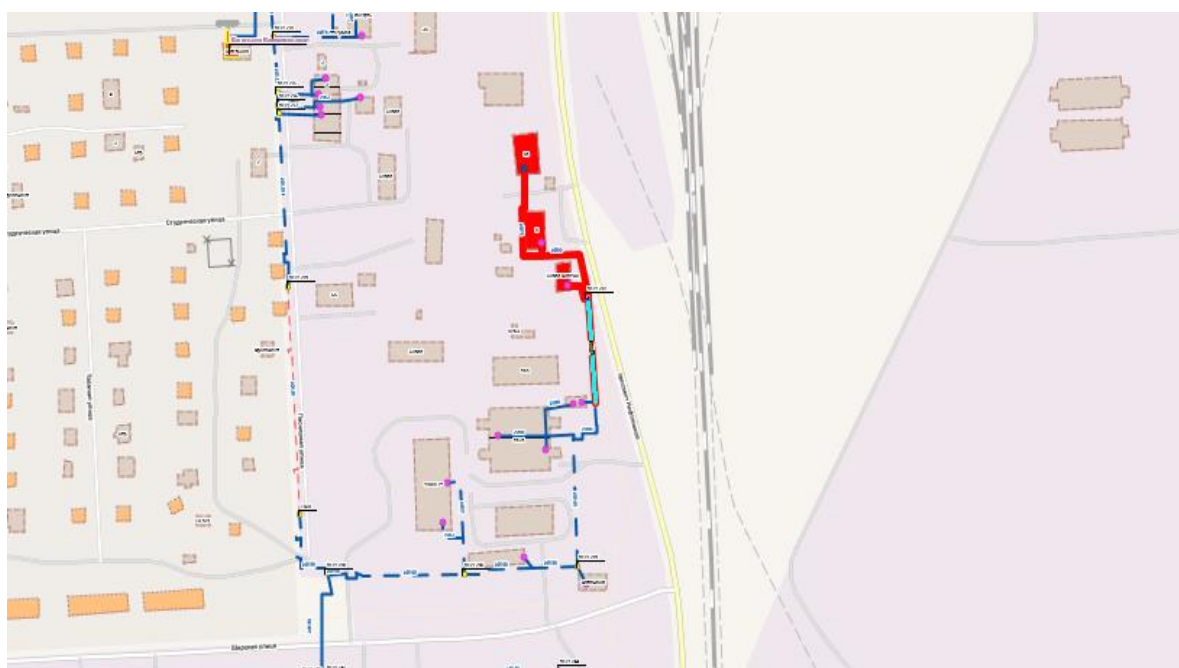
Рисунок 33. Визуализация отключения запорной арматуры ЗУ Уз.103-«Регион груз сервис» (котельная по ул. Комсомольская)
