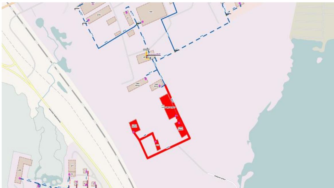
Рисунок 36. Визуализация отключения запорной арматуры Уз.483- Уз.482 (котельная КСАТ)
