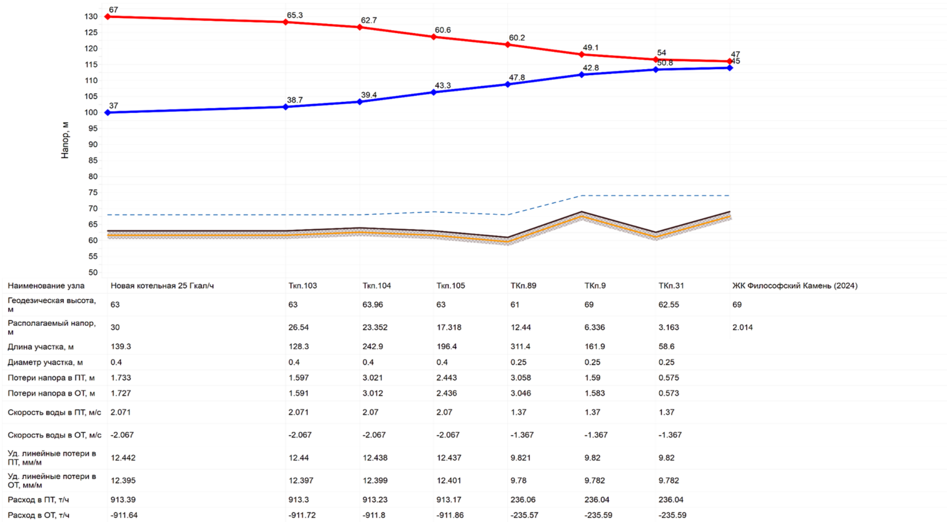
Рисунок 10. Пьезометрический график участка сети от Котельной 25 Гкал/ч до ЖК «Философский камень»
