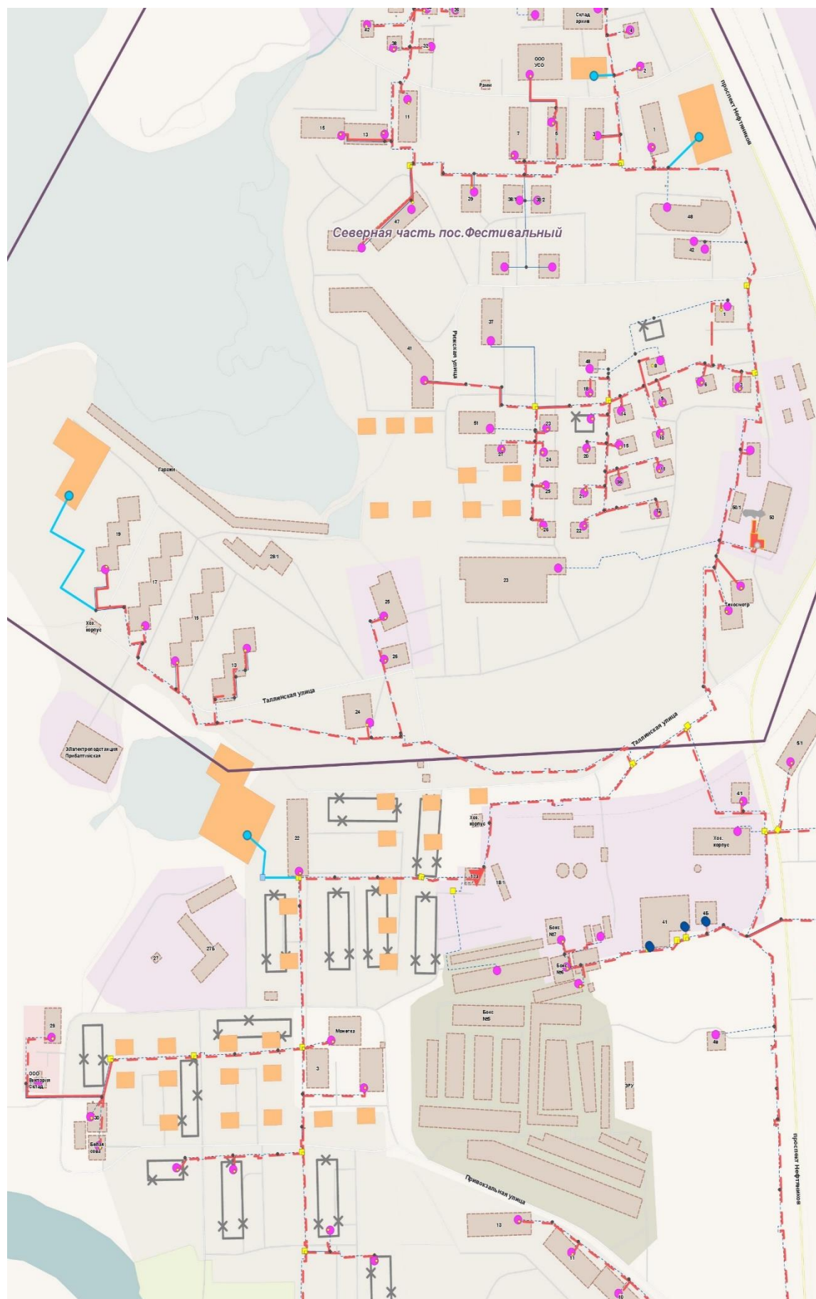
Рисунок 25. Схема подключения перспективных объектов северная часть п. Фестивальный
