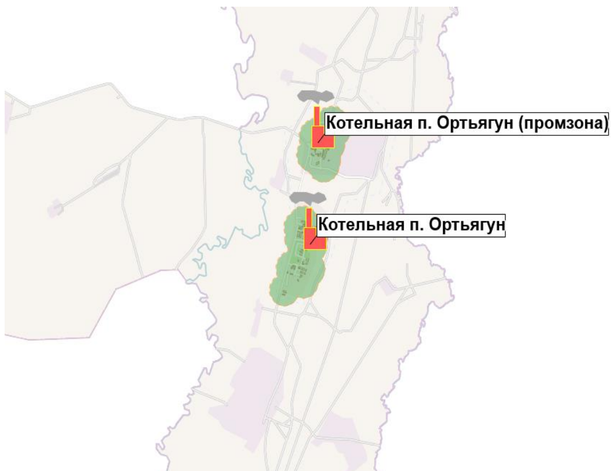
Рисунок 7. Ориентировочные зоны радиусов эффективного теплоснабжения для средне подключаемой тепловой нагрузки к точкам сброса
