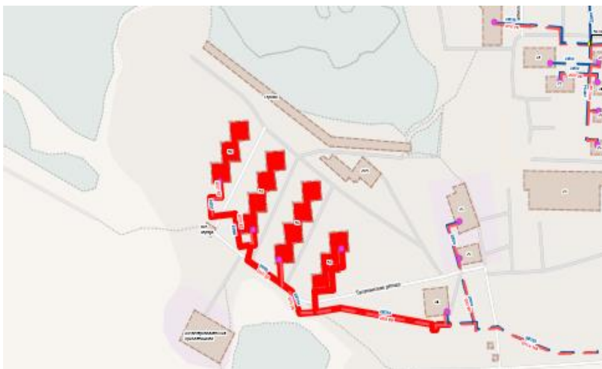
Рисунок 37. Визуализация отключения запорной арматуры Уз.564-19УТ-70 (Котельная ПМК-177)
