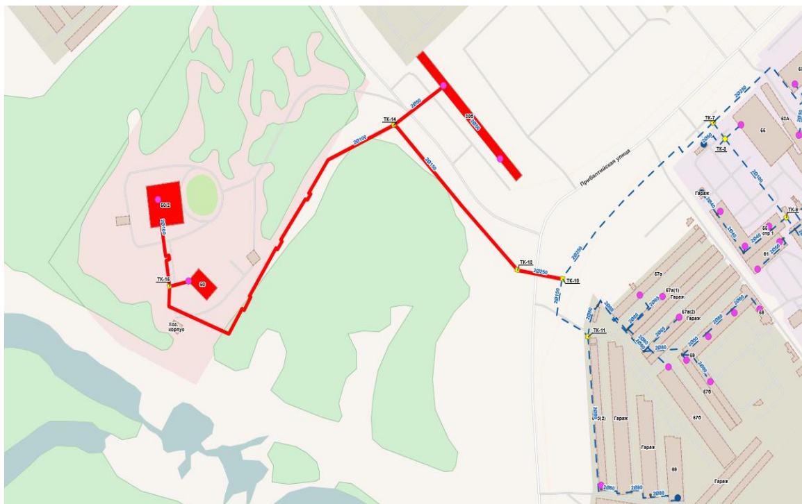
Рисунок 32. Визуализация отключения запорной арматуры ЗУ Уз.103-«Регион груз сервис» (котельные коммунальной зоны)
