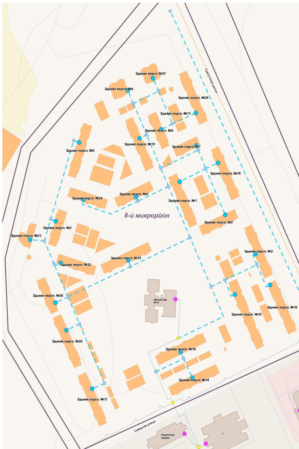
Рисунок 15. Схема подключения перспективных объектов в 8 мкр.
