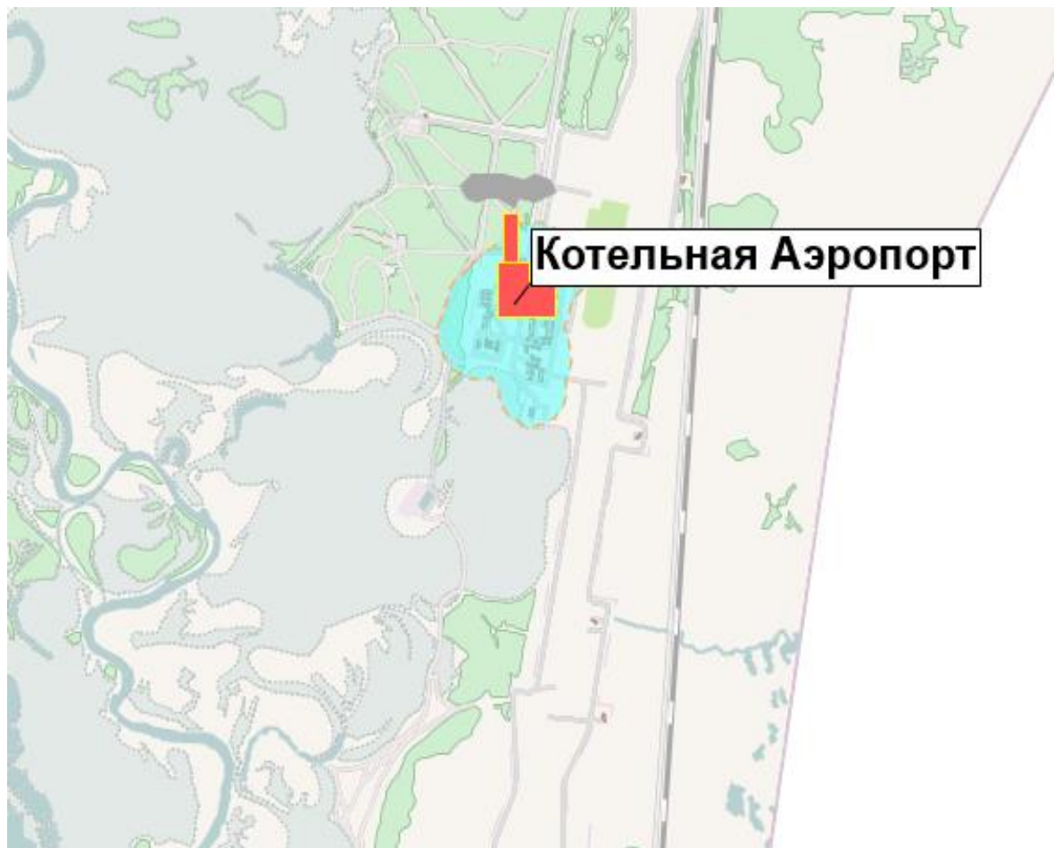
Рисунок 8. Ориентировочные зоны радиусов эффективного теплоснабжения для средне подключаемой тепловой нагрузки к точкам сброса
