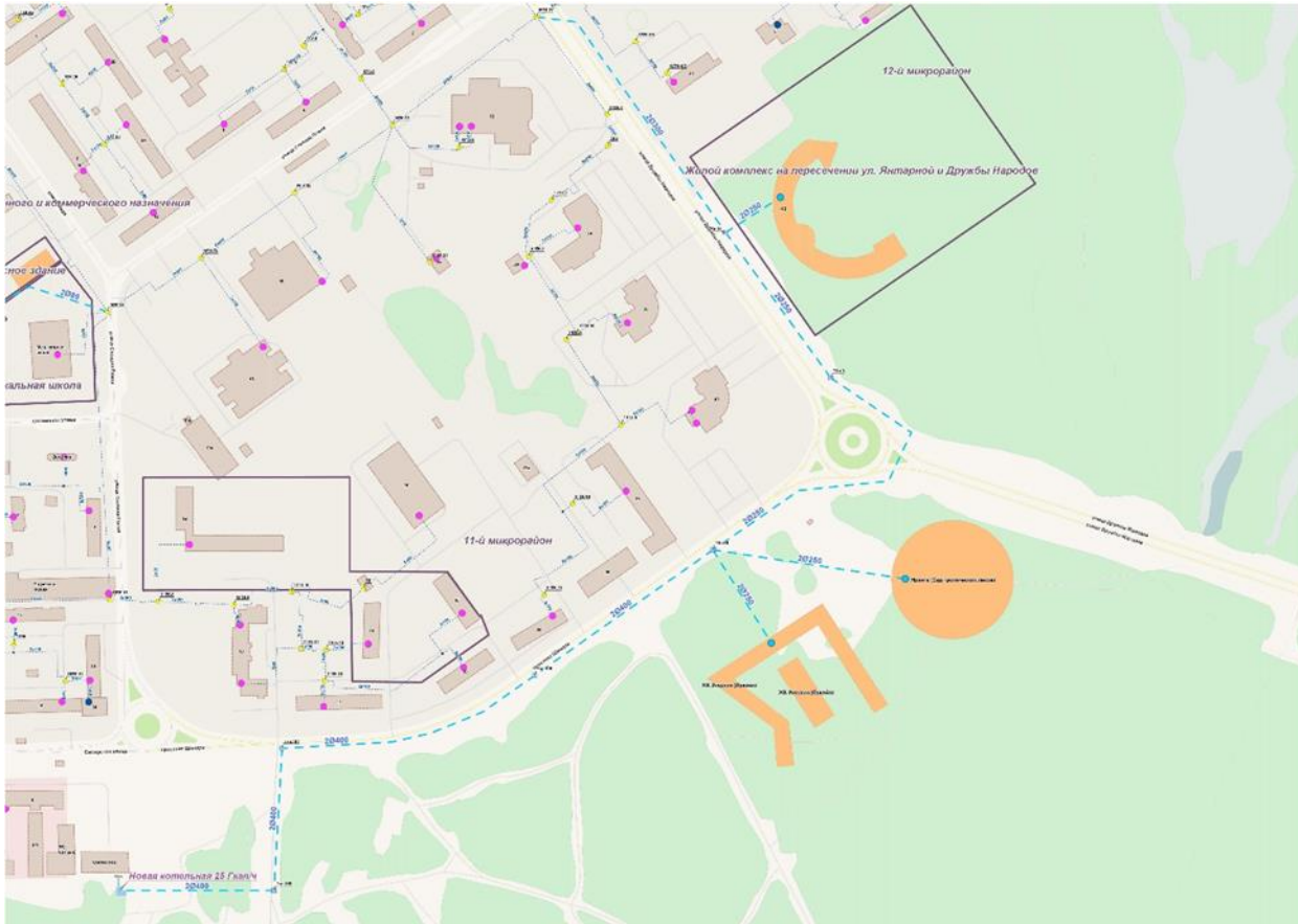
Рисунок 9. Схема подключения перспективных абонентов на основании Варианта №1
