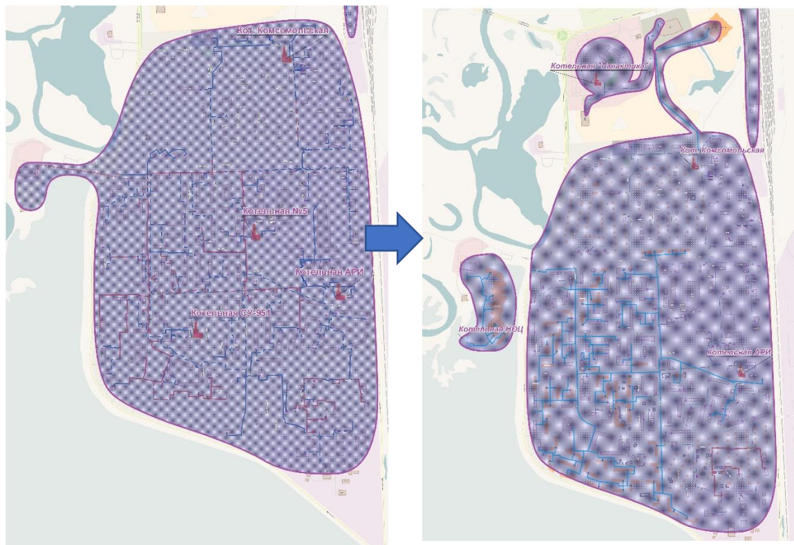
Рисунок 13. Зоны действия существующих котельных № 5, № 1 (Арочник) и № 2 (СУ-951) и новой котельной № 1 (Арочник) мощностью 53,4 МВт
