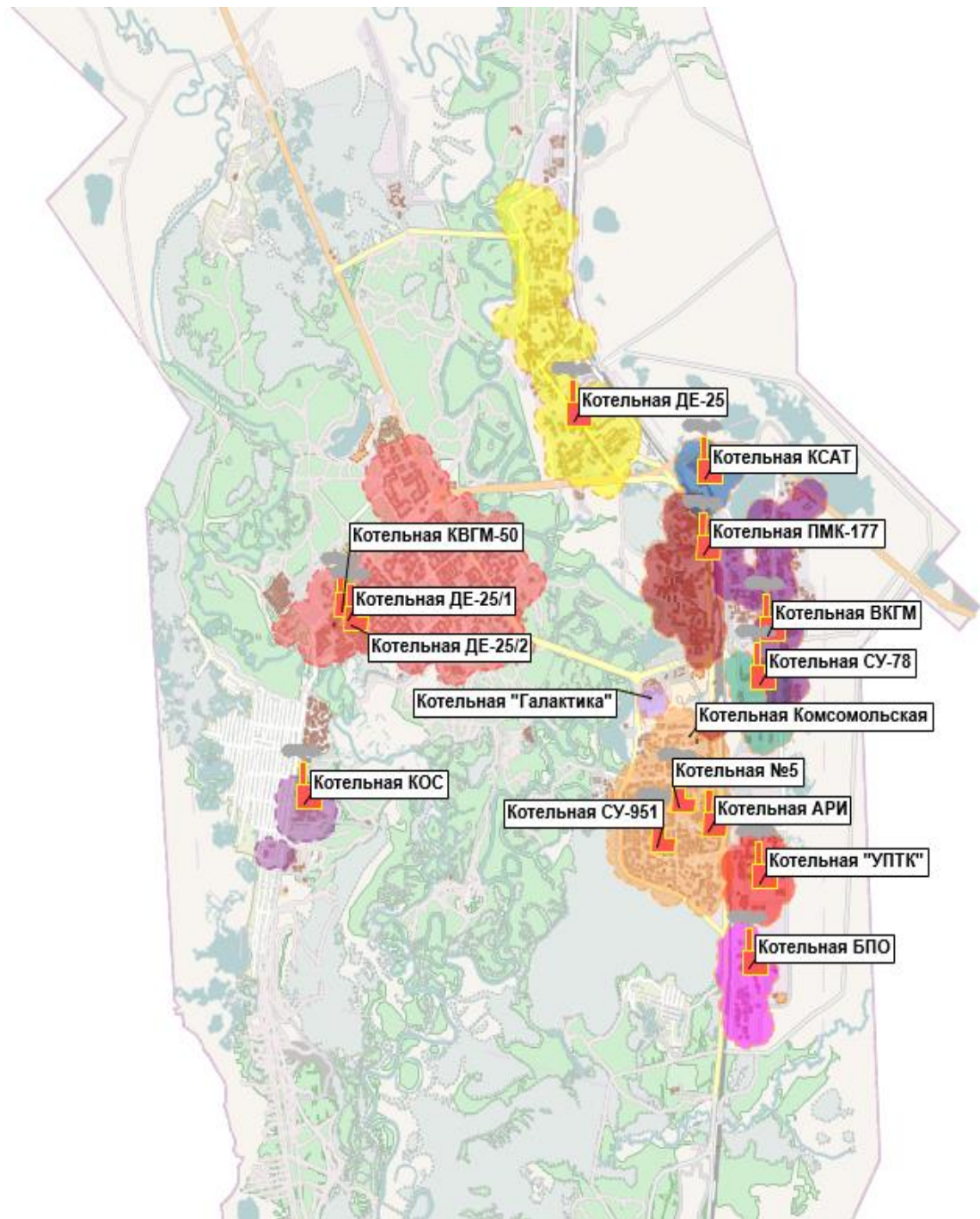
Рисунок 6. Ориентировочные зоны радиусов эффективного теплоснабжения для средне подключаемой тепловой нагрузки к точкам сброса
