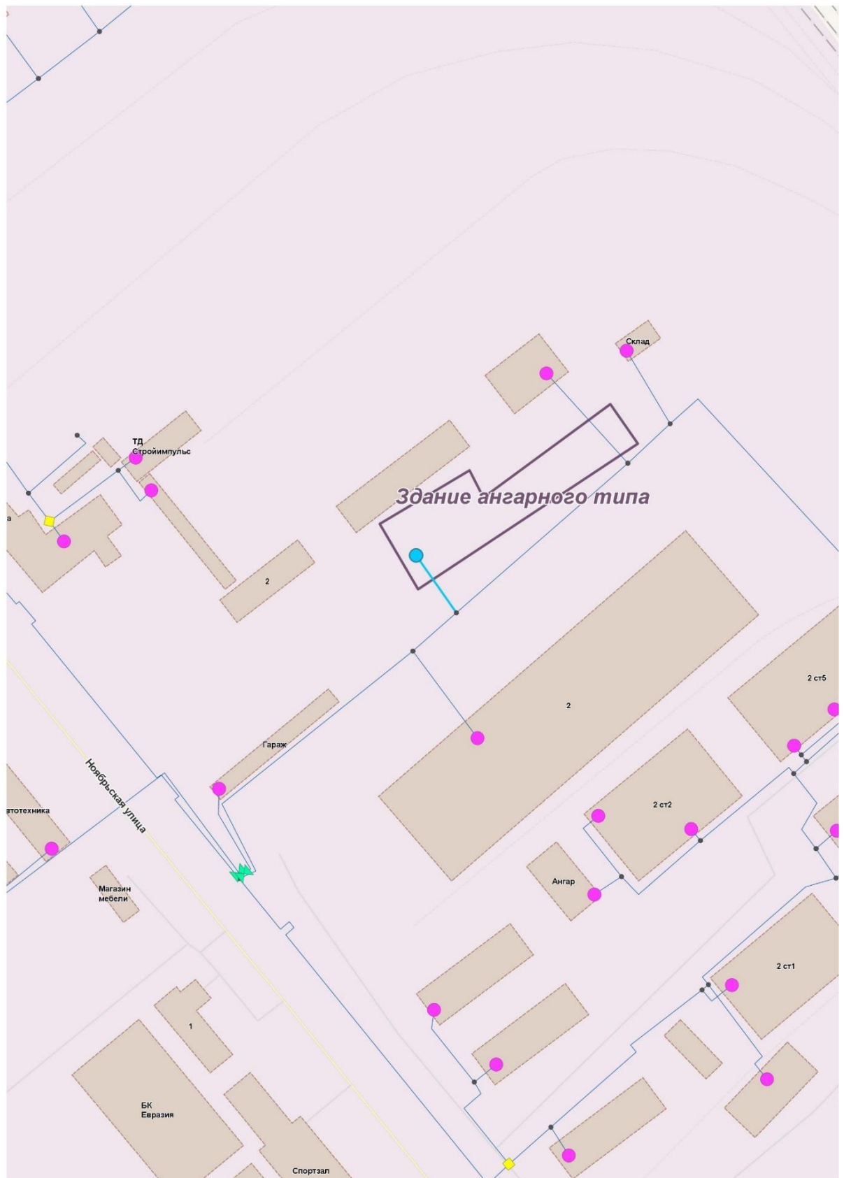
Рисунок 20. Схема подключения перспективного потребителя «Здание ангарного типа»
