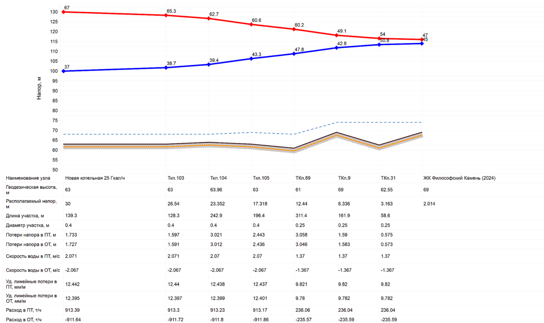
Рисунок 10. Пьезометрический график участка сети от Котельной 25 Гкал/ч до ЖК «Философский камень»
