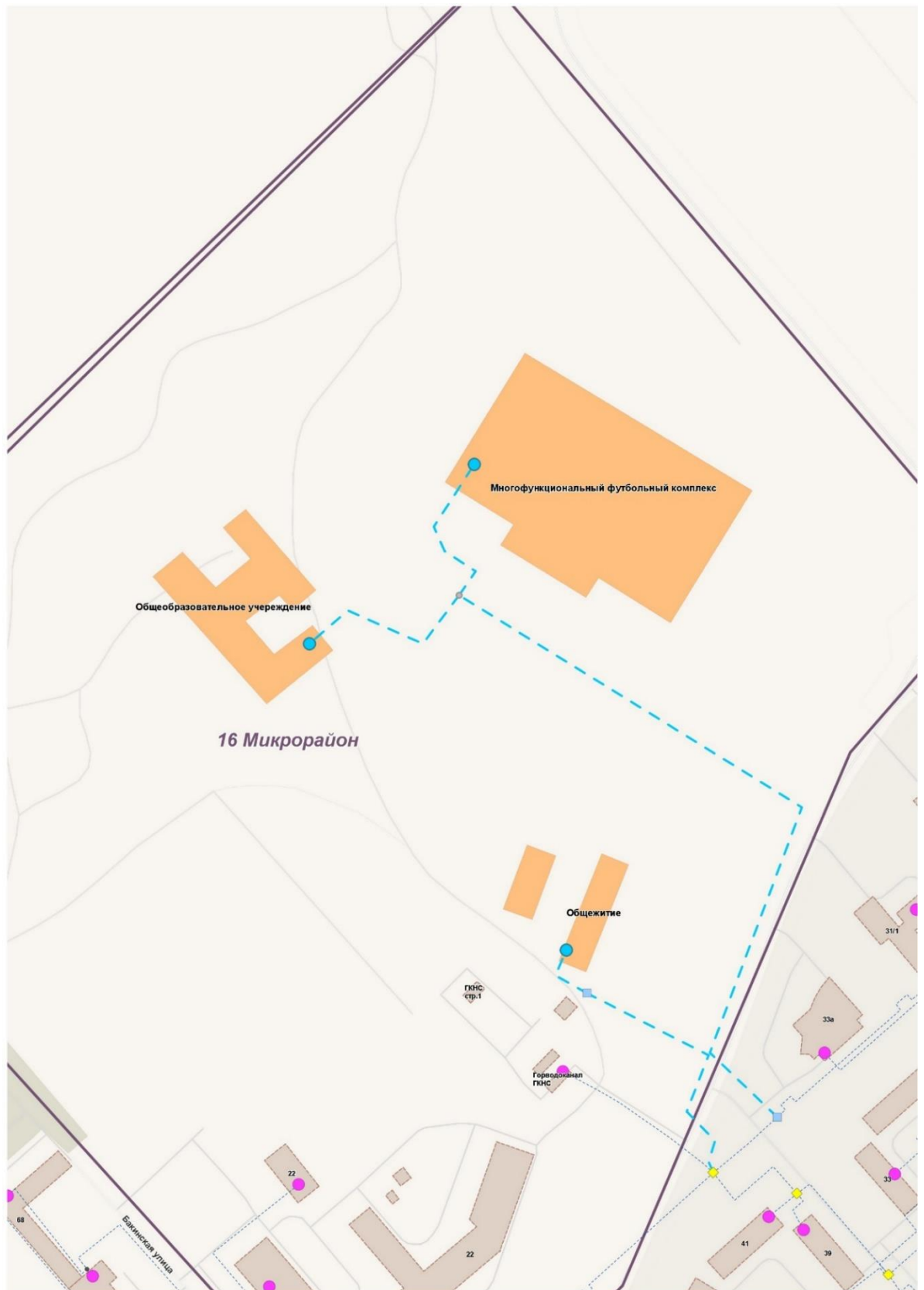
Рисунок 16. Схема подключения перспективных объектов в 16 мкр.
