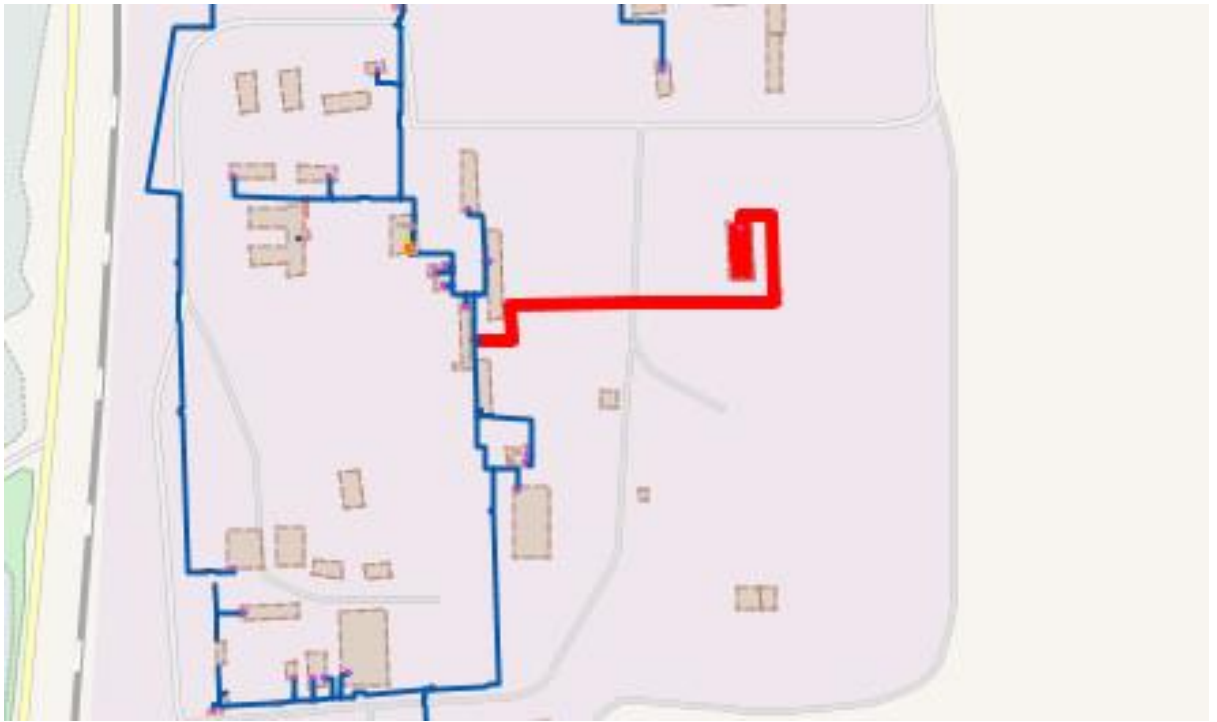
Рисунок 28. Визуализация отключения запорной арматуры ЗУ Уз.298- Уз.298 (котельная БПО)
