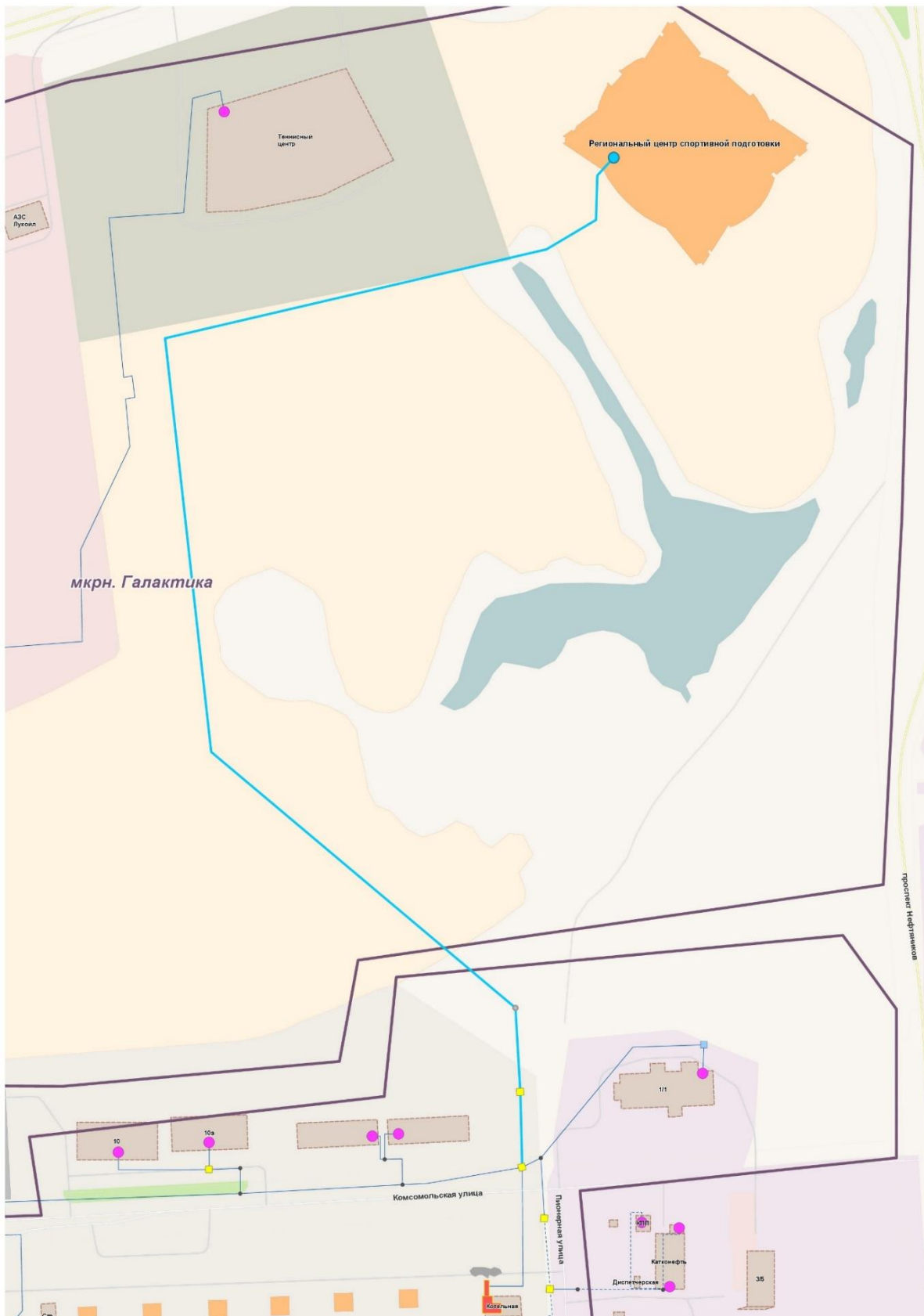
Рисунок 21. Схема подключения перспективного потребителя «Региональный спортивный центр»
