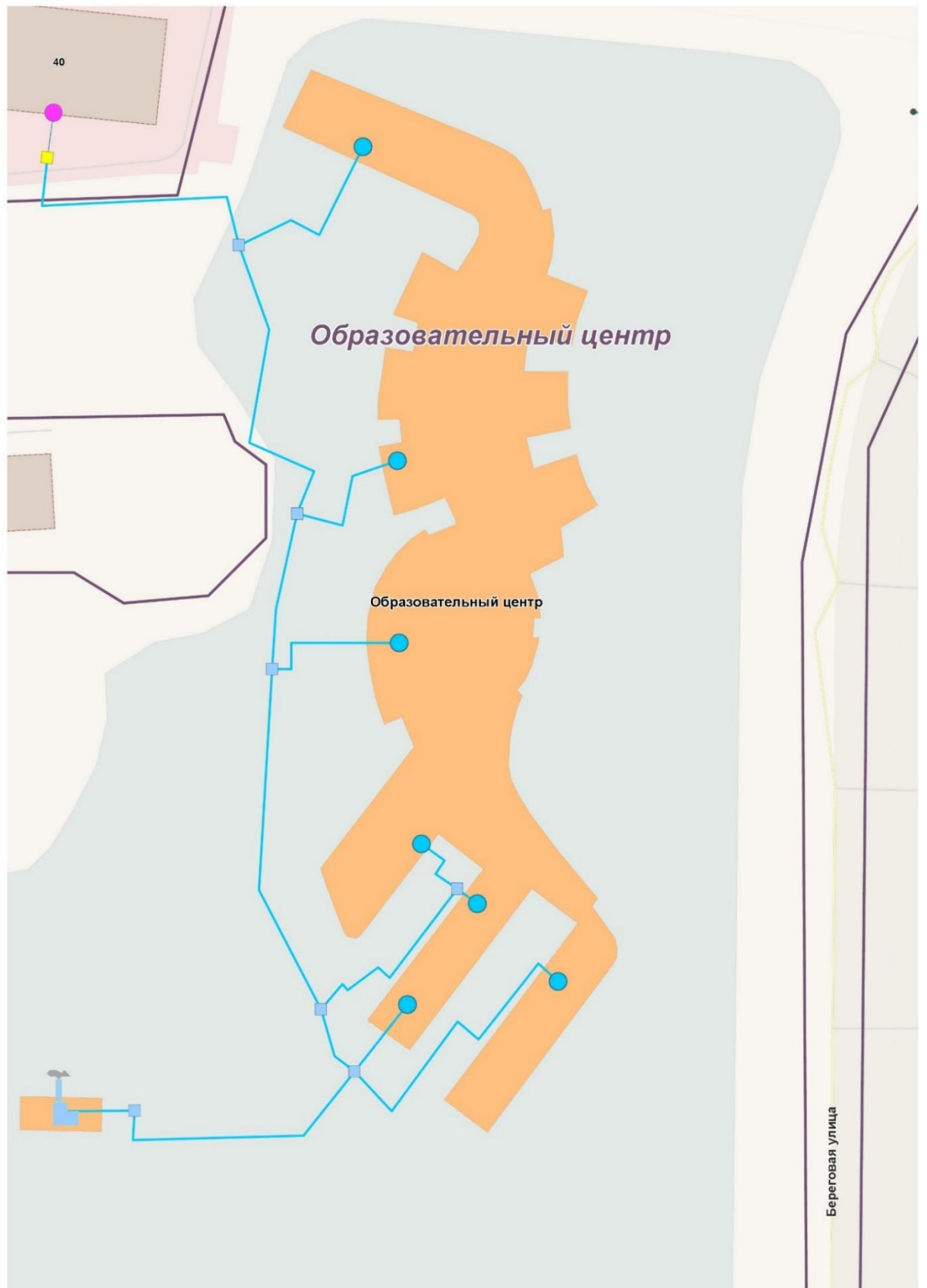
Рисунок 22. Схема подключения перспективного потребителя «Научно-образовательный центр»
