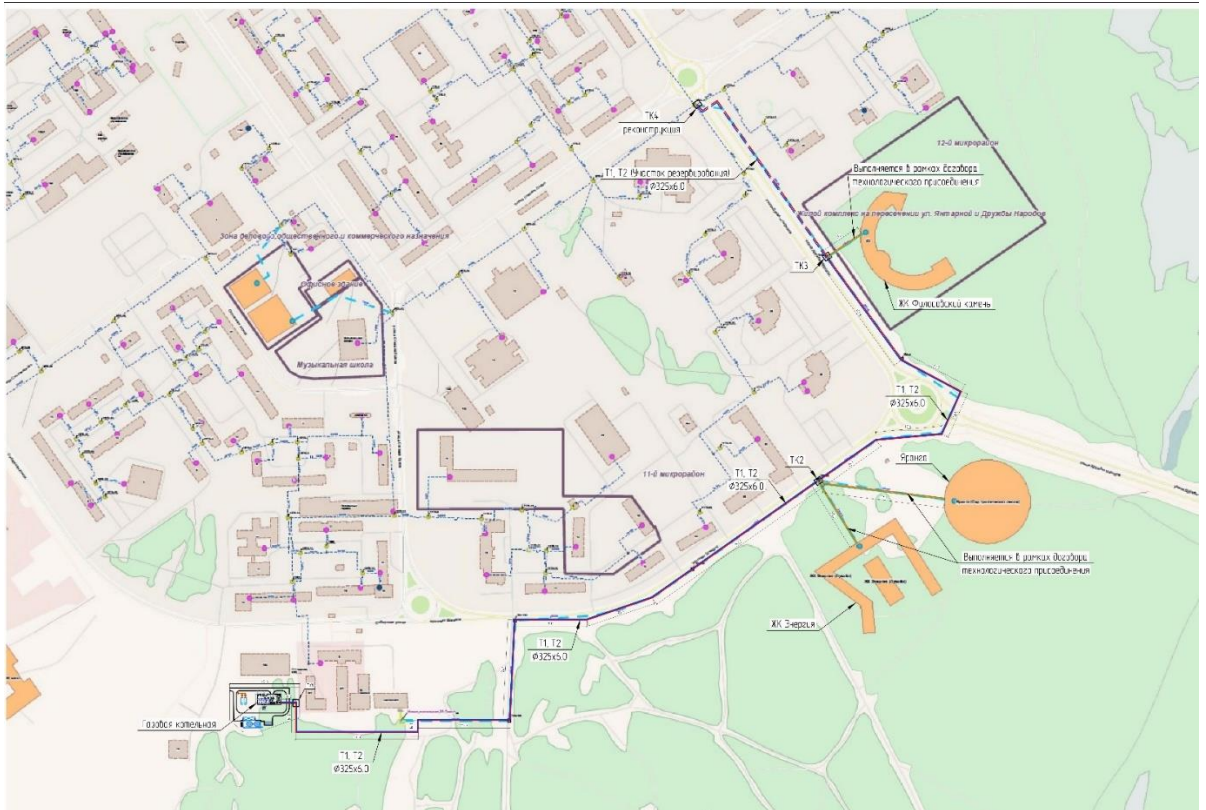
Рисунок 9. Схема подключения перспективных абонентов на основании Варианта №1
