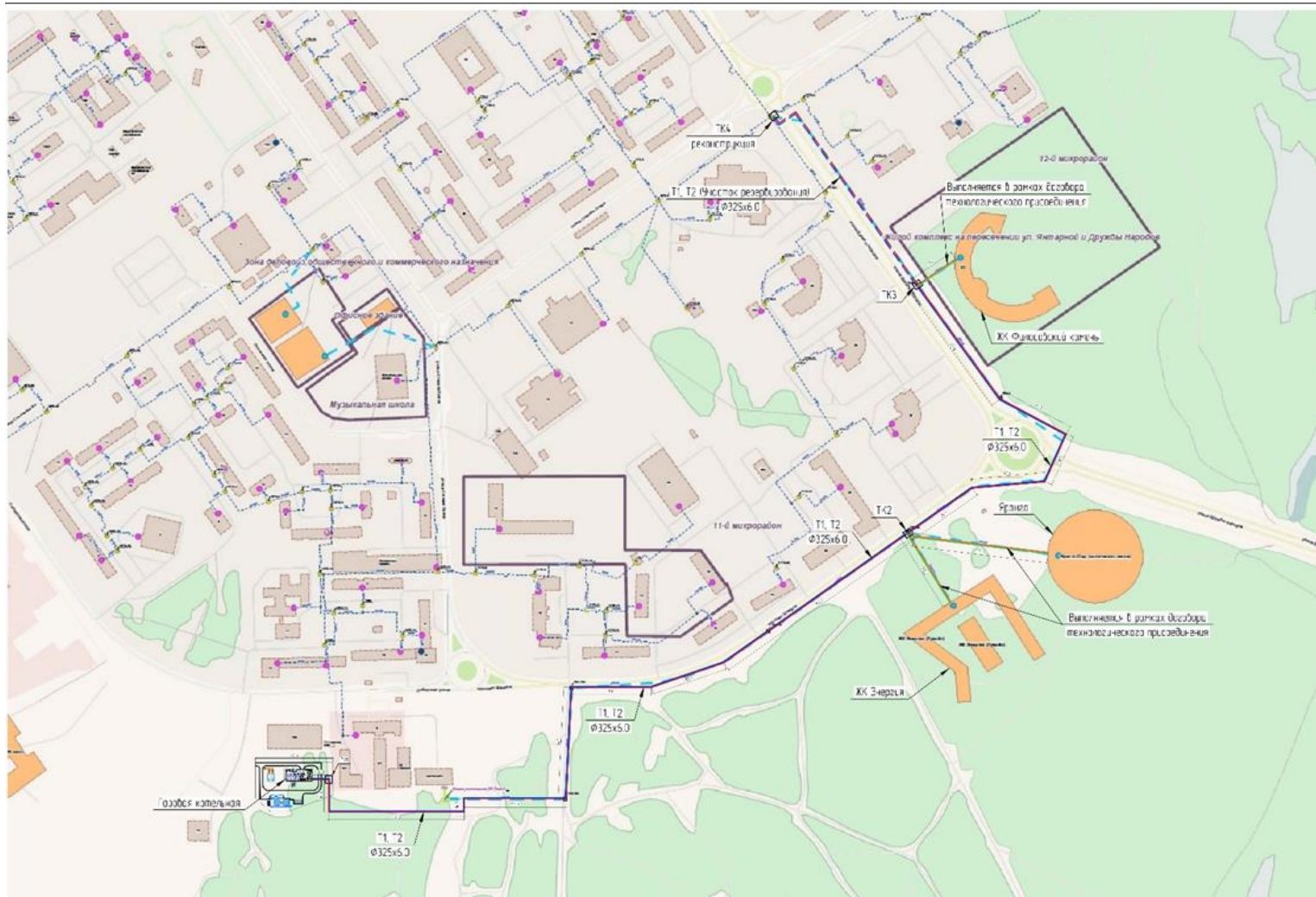
Рисунок 14. Схема подключения перспективного потребителя «Жилой комплекс Философский камень», ЖК «Энергия» и сад тропических лесов (Яранга)
