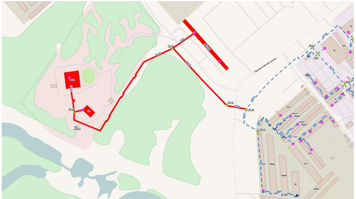
Рисунок 32. Визуализация отключения запорной арматуры ЗУ Уз.103-«Регион груз сервис» (котельные коммунальной зоны)
